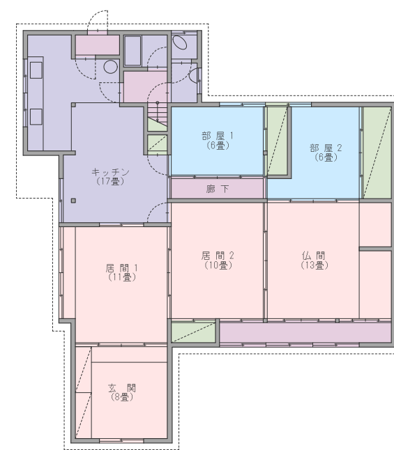
【1階平面図 1/200】
